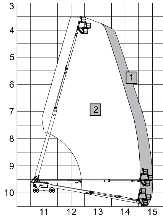
SX-125 XC Diagram over bevegelsesområde
