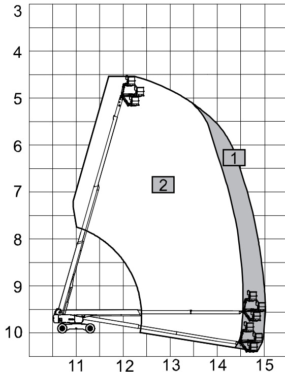
SX-105 XC Diagram over bevegelsesområde
